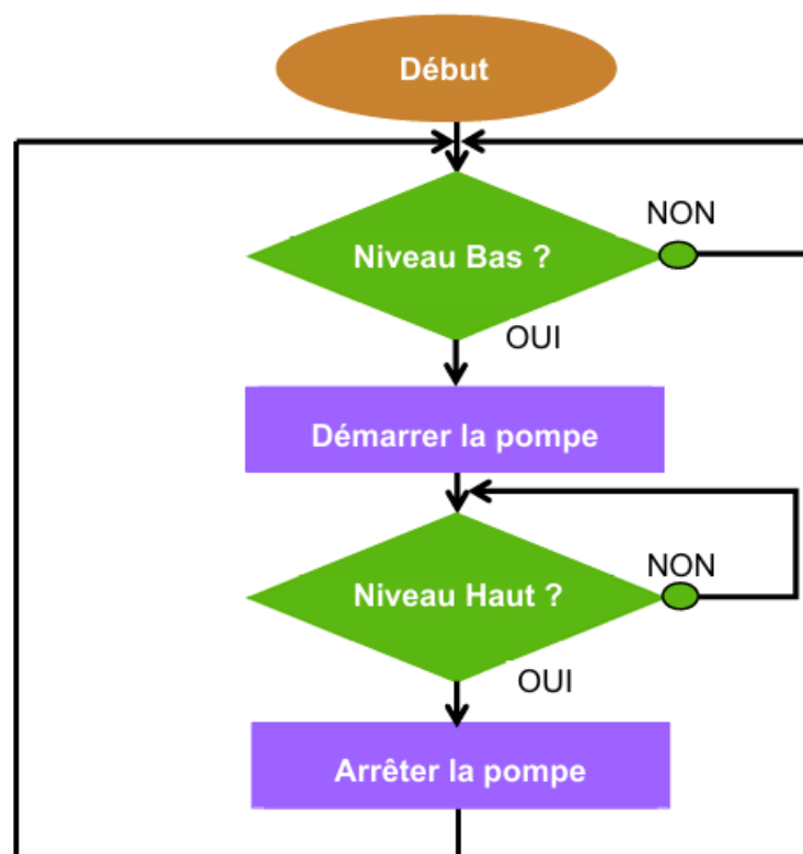
Figure 4 : algorithme du fonctionnement de la pompe
