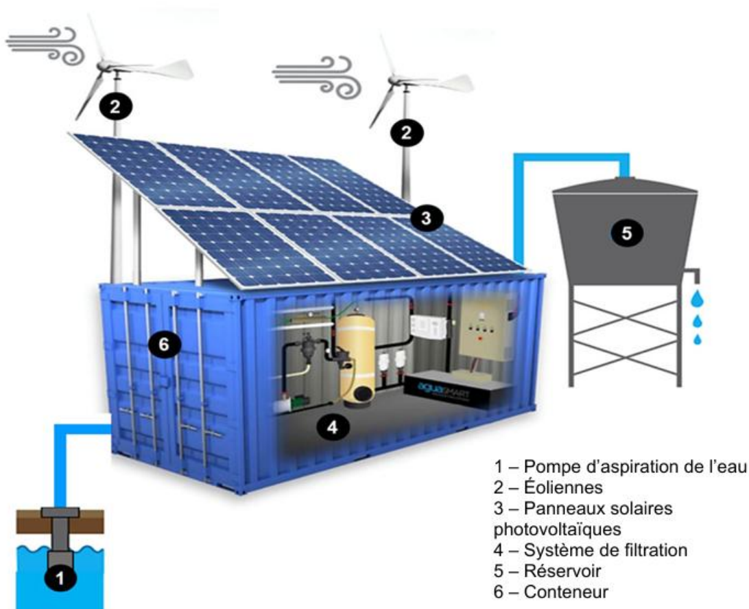
Figure 1 : schéma descriptif du système
